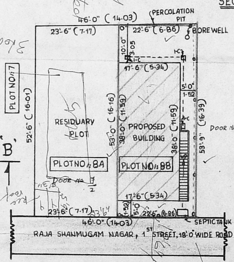
SUB-DIVISION SITE PLAN
